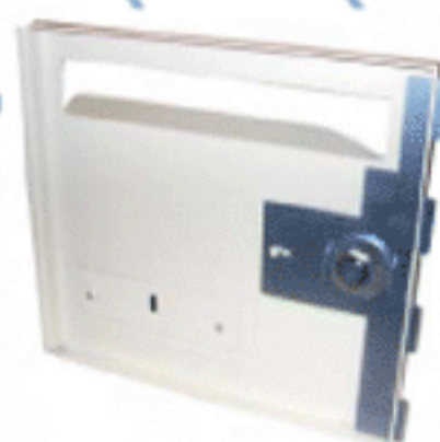
Portillon Gamma 34 Antivandale - Acier Ep.2mm avec système translatif 4 points
